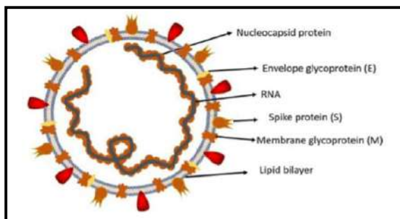
Gambar 1. 2. Struktur Coronavirus
